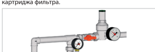
Установка на горизонтальном трубопроводе
